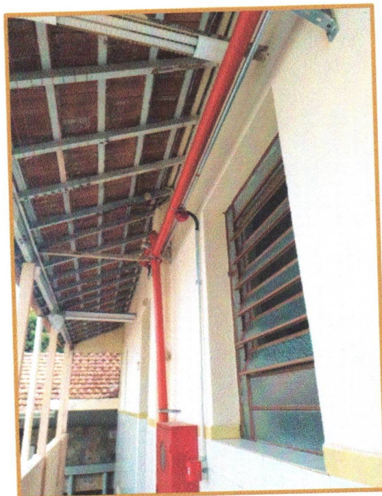
Rede de Alarme de Incêndio
