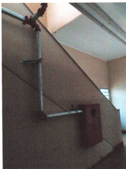
Hidrante Piso Térreo CDHU
